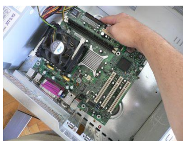
Figura 2.2. 4.1 Instalarea plăcii de bază în carcasă
