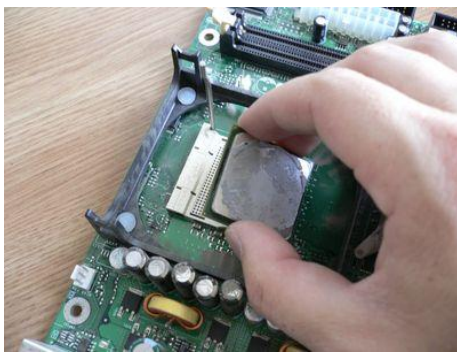
Figura 2.2.1 Instalarea procesorului pe placa de bază
